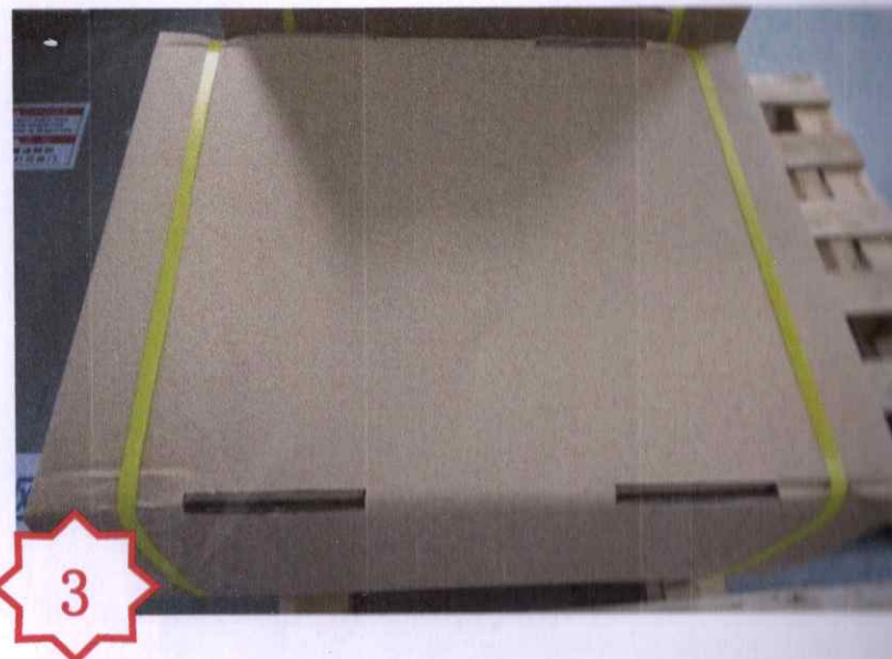
图三，确认 PA914 无漏装后，将 26 的内箱与外箱配合后，并打包装带待出货。
